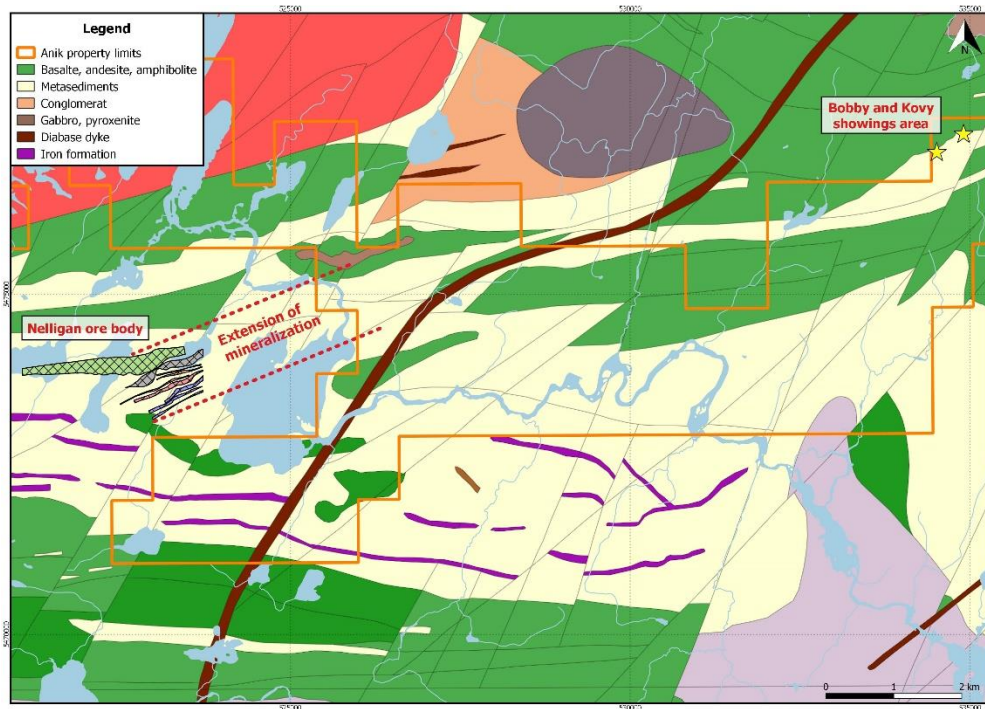
Figure 2: Propriété Anik - géologie régionale
