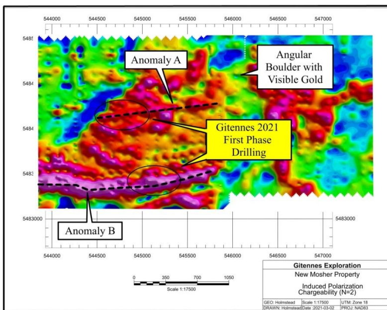
Figure 1: New Mosher - Chargeabilité PP élevée (représentée en rose) et secteurs prioritaires.
