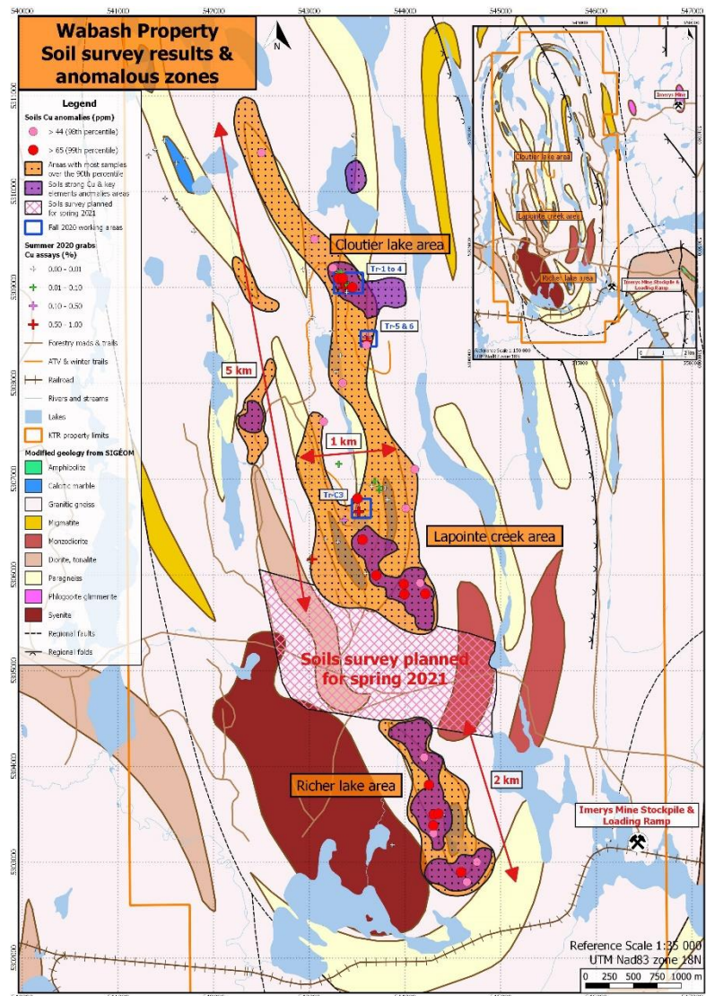
Figure 1: Wabash – anomalies géochimiques
