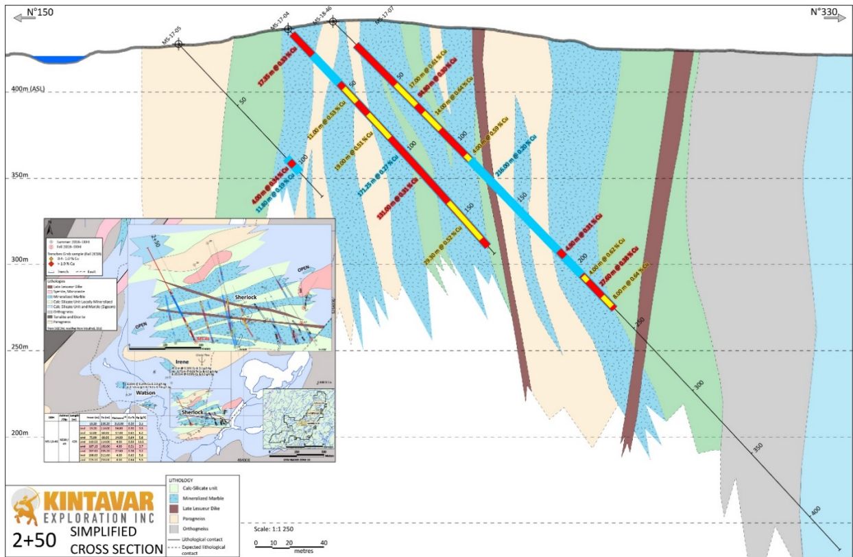
Figure 1: Coupe transversale 2 +50 pour la zone de Sherlock. La figure pleine résolution peut être téléchargée ici.
